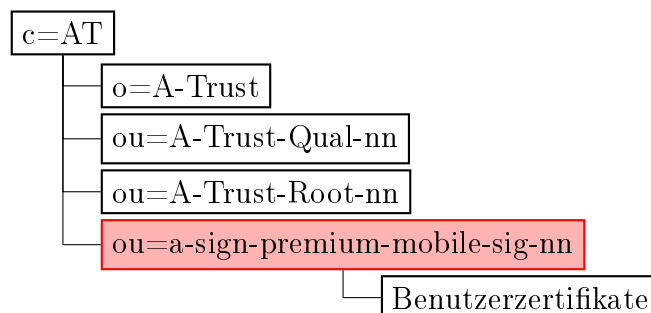
Abbildung 2: A-Trust Verzeichnisbaum
