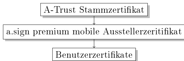
Abbildung 1: Zertifikatshierarchie
